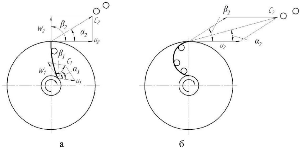
Рис. 1. Схема руху частинок льоду при кріогенному бластингу а – радіальне розташування направляючих жолобів ( \beta_1=90^\circ ); б – жолоби загнуті вперед у напрямку обертання ( \beta_1<90^\circ );
