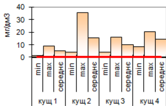
г) Залізо (загальне)
