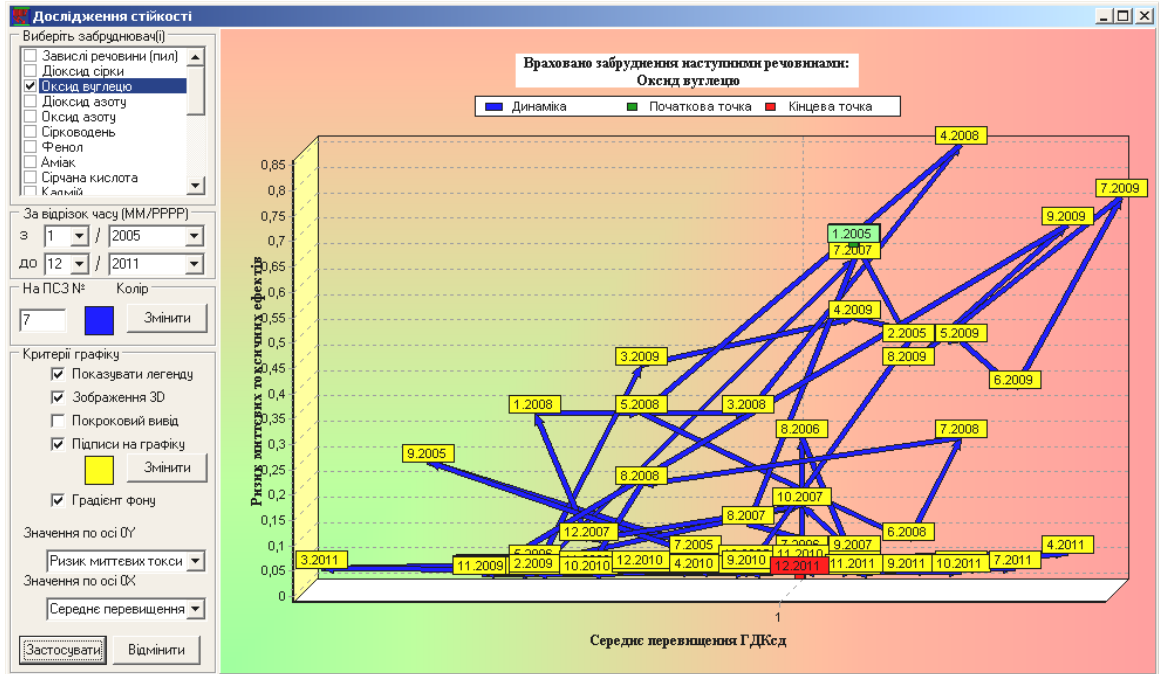
Рис. 7. Динаміка впливу оксиду вуглецю на ПСЗ №7 (2005 – 2011).
