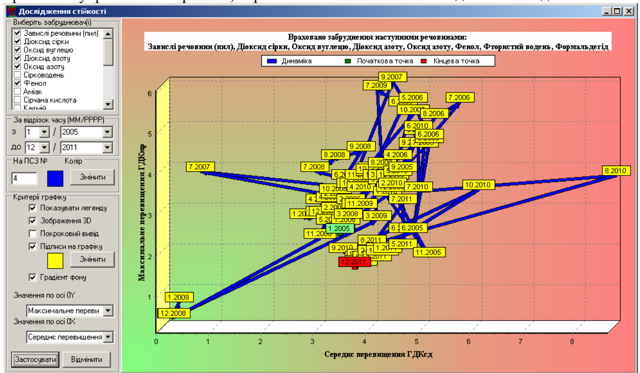
Рис. 4. Моніторинг динаміки техногенного впливу за індексом ІЗА
